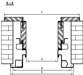
D - szerokość otworu montażowego
