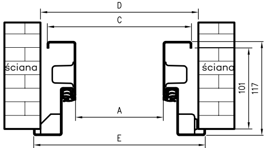
Przekrój poprzeczny ościeżnicy w murze
