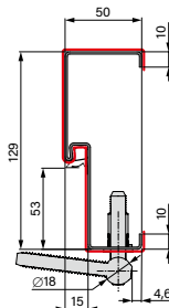
OŚCIEŻNICA STALOWA
