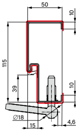
OŚCIEŻNICA STALOWA
