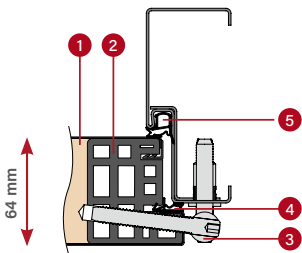
OŚCIEŻNICA STAŁOWA
