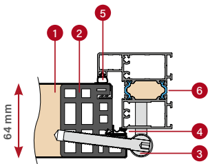
OŚCIEŻNICA ALUMINIOWA
