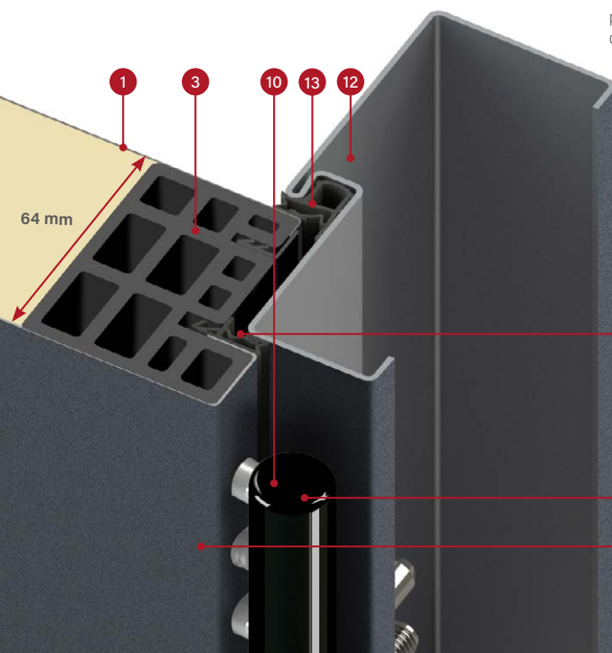
przekrój ościeznicy stalowej dla skrzydła THERMO 64
