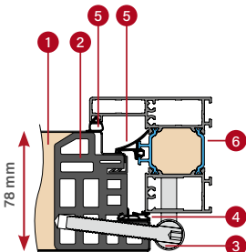
OŚCIEŻNICA ALUMINIOWA
