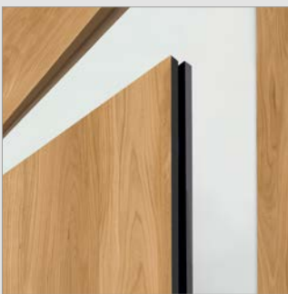
Panel środkowy wykonany z płyty barwionej w kolorze czarnym, felc panelu nie posiada obrzeża, front panelu pokryty dekiem zgodnie z kolorystyką skrzydła
